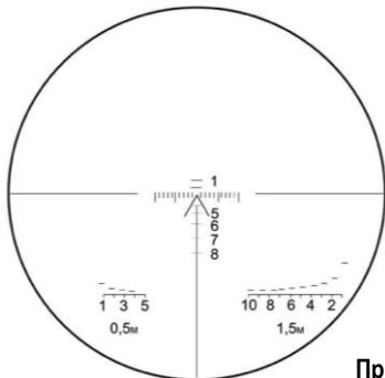
Прицельная сетка с шкалами измерения дальности
